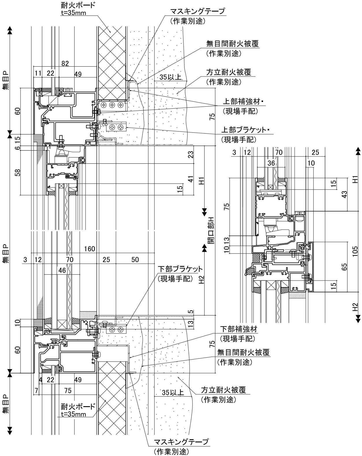
■【防火(個別)】Lタイプ カーテンウォール仕様 160見込(複層) たてすべり出し窓/FIX段窓部(複層内網・36溝障子) 縦断面図
